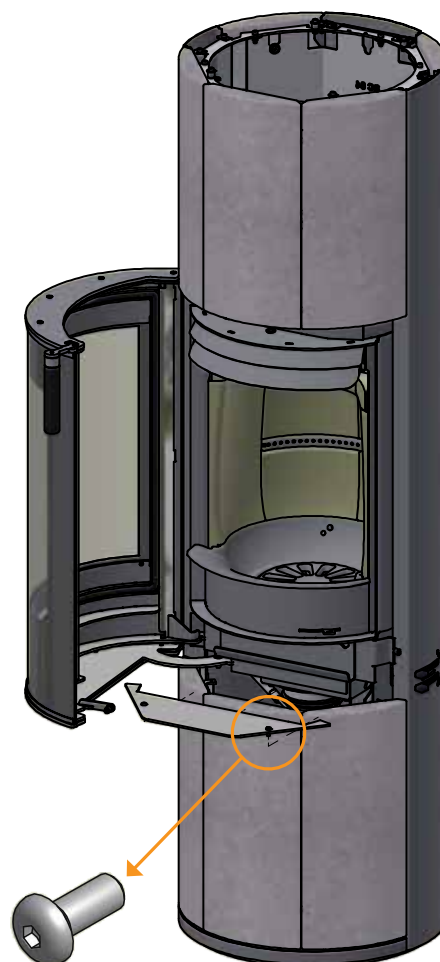
2 Inbusschrauben M5x12 RH
