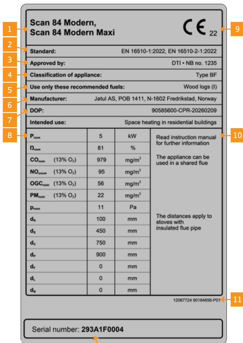
Typenschild
